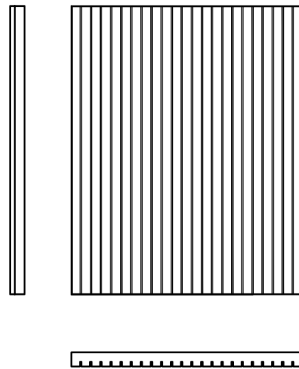
A4. Anta con tamponamenti in legno cannettato
